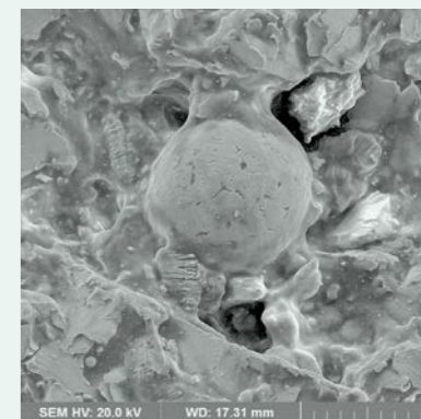
Оксидное включение в изломе образца сварного шва
