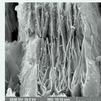
Слоистая структура вермикулита на поперечном сечении
